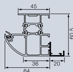
Eenzijdige verbreding
