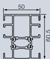
Verbreidingsprofiel 50 mm
