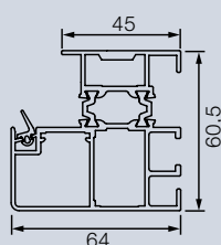
Kozijn A2
