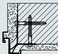
Inbouw met plugankers
