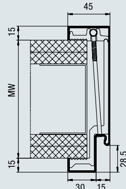
Profiel 21120 Klauenbevestiging
