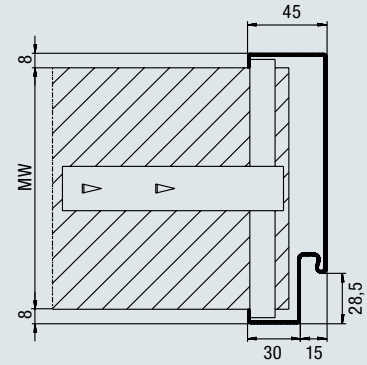
Profiel 21101
