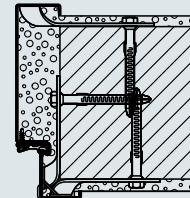
Hoekkozijn met aanvullend kozijn Inbouw met plugankers
