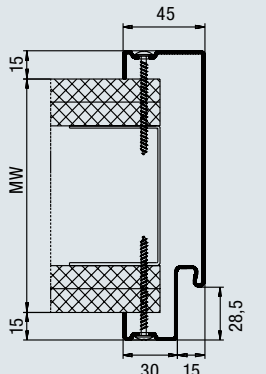
Profiel 21120 Spiegelschroefbevestiging
